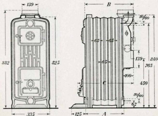
DIMENSIONS PRINCIPALES
