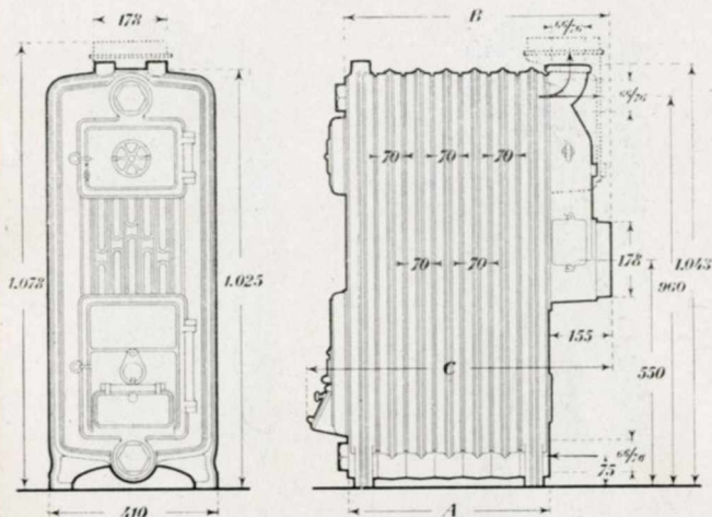
DIMENSIONS PRINCIPALES
