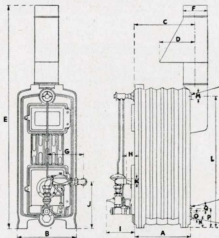
DIMENSIONS PRINCIPALES
