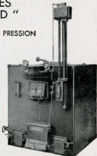
avec régulateur hydrostatique
