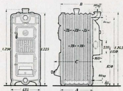
DIMENSIONS PRINCIPALES
