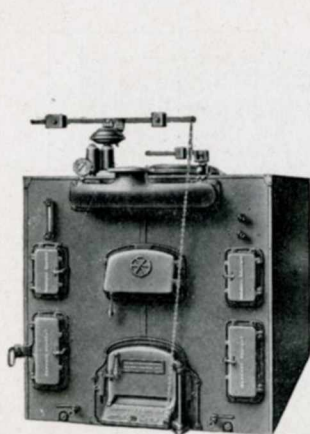
avec régulateur à poche
