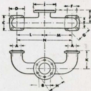
Chaudières A-5, A-6 et D-2
