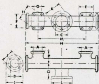
Chaudières A-4, A-5, A-6 et D-2 à 3 retours
