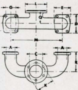
Chaudière D à 1 retour
